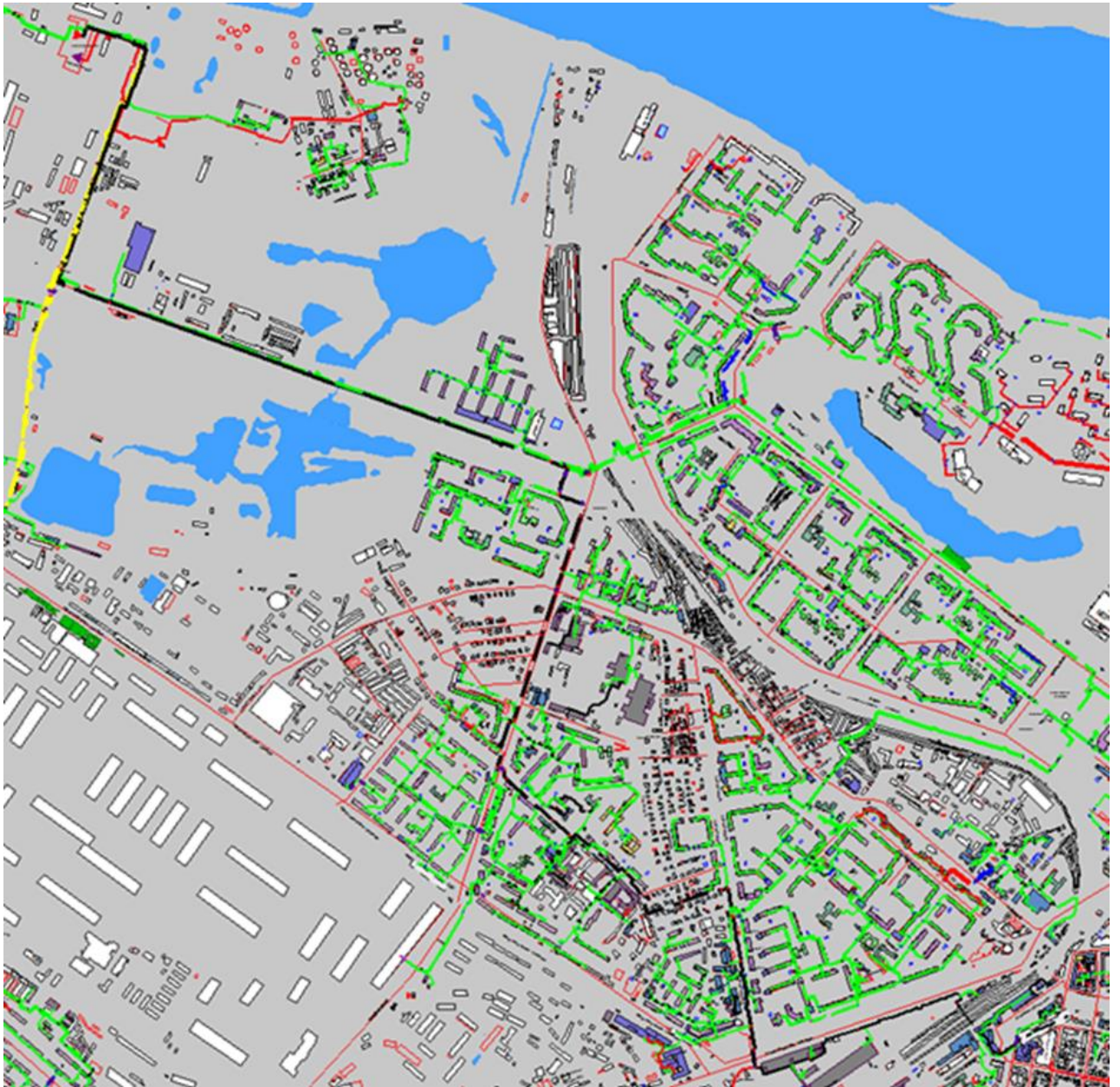
Рисунок 3.4 – Трассировка теплопровода от Сормовской ТЭЦ до конечного потребителя «ПТ-пл.Револ,7 вест2»
