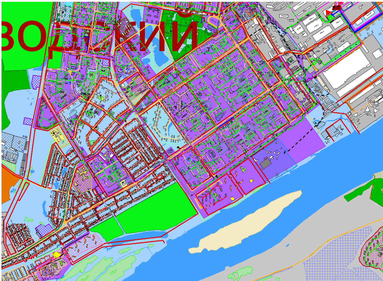
Рисунок 3.16 – Трассировка теплопровода от Авозаводской ТЭЦ до конечного потребителя «ПТ-Пилотов,21а»
